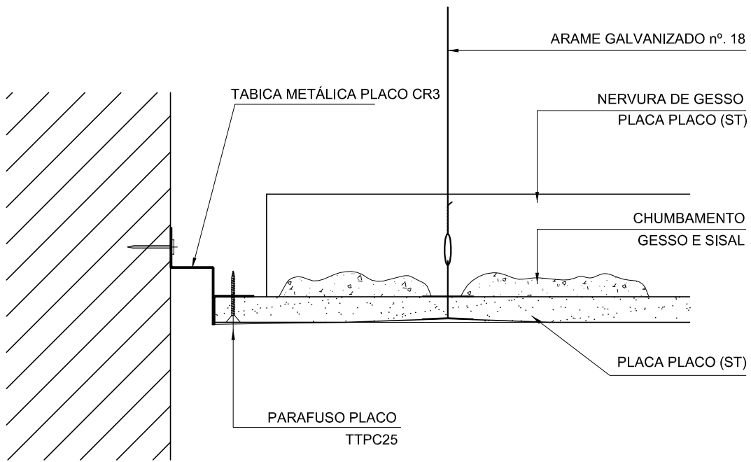
CORTE TRANSVERSAL ÀS PLACAS
