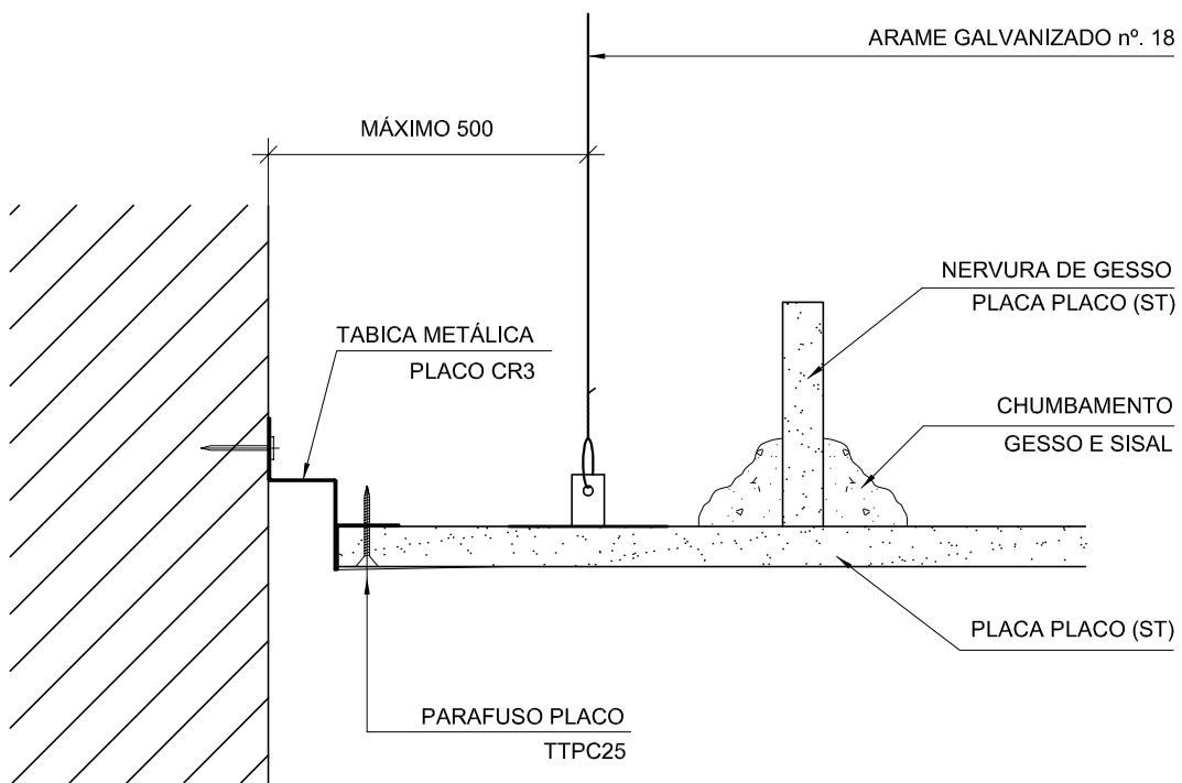
CORTE LONGITUDINAL ÀS PLACAS
