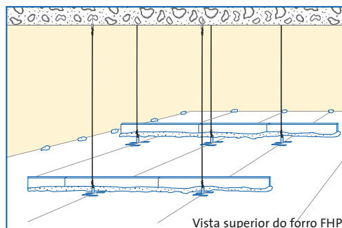
Vista superior do forro FHP
